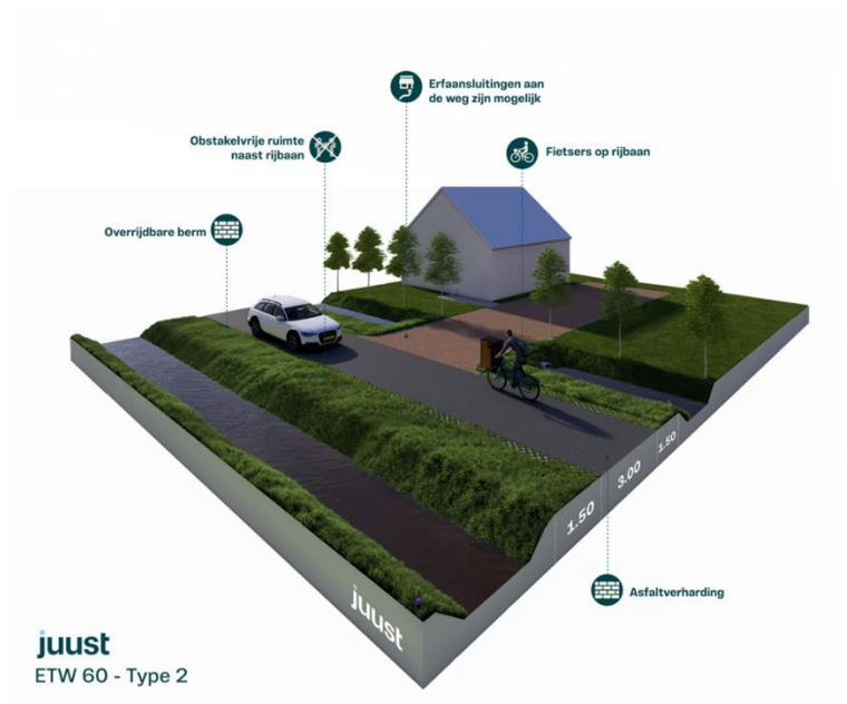
Figuur 9: Profiel ETW(60) type 2
